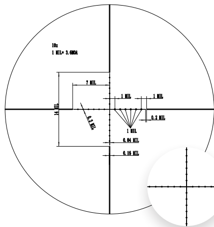
Mil-Dot
