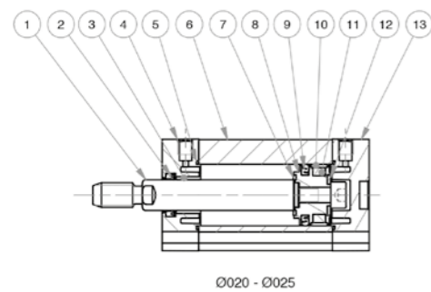
Ø020 - Ø025
