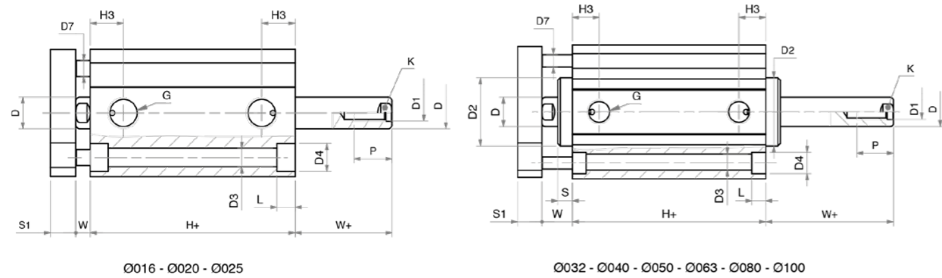
Model FDPA, FDMPA
