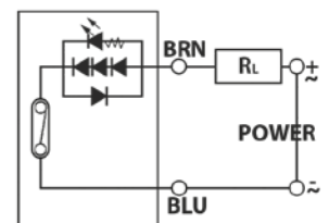
2-polig rechte bouwvorm
