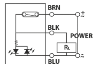
3-polig rechte bouwvorm
