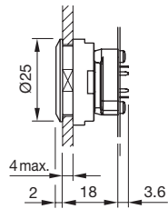
PCB 款式
