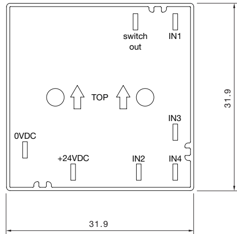
组件布局
