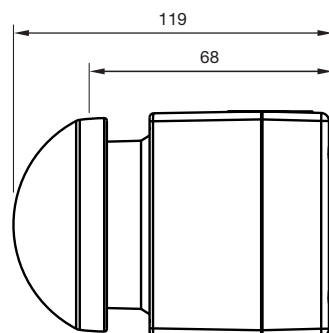
Slagdrukknop
