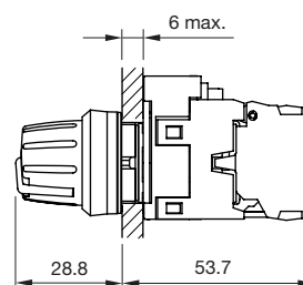
Keuzeschakelaar ronde hendel
