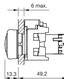
Drukknop/verlichte drukknop
