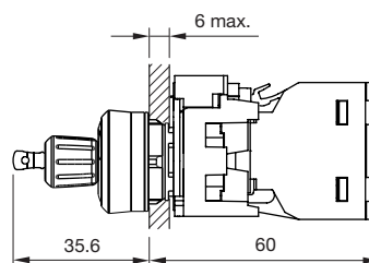
ID-sleutelschakelaar
