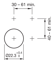
Montagegaten opbouwuitvoering
