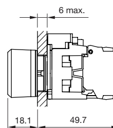
Drukknop/verlichte drukknop
