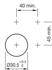
Montagegaten inbouwuitvoering
