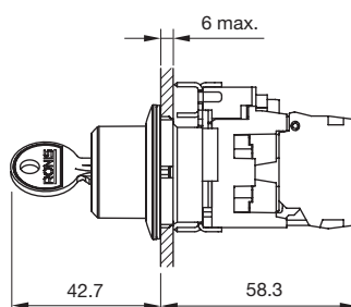
Keuzeschakelaar
