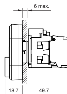
Dubbele drukknop
