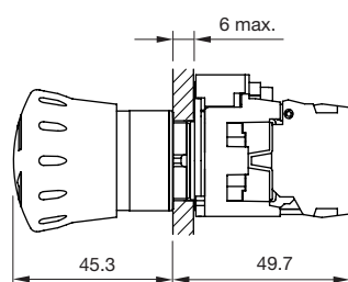
Slagdrukknop
