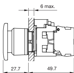
Paddenstoeldrukknop
