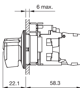
Afmetingen opbouwuitvoering Signaalarmatuur
