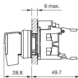
Potentiometer
