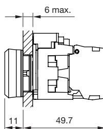
Afmetingen opbouwuitvoering Signaalarmatuur
