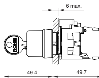
ID-sleutelschakelaar
