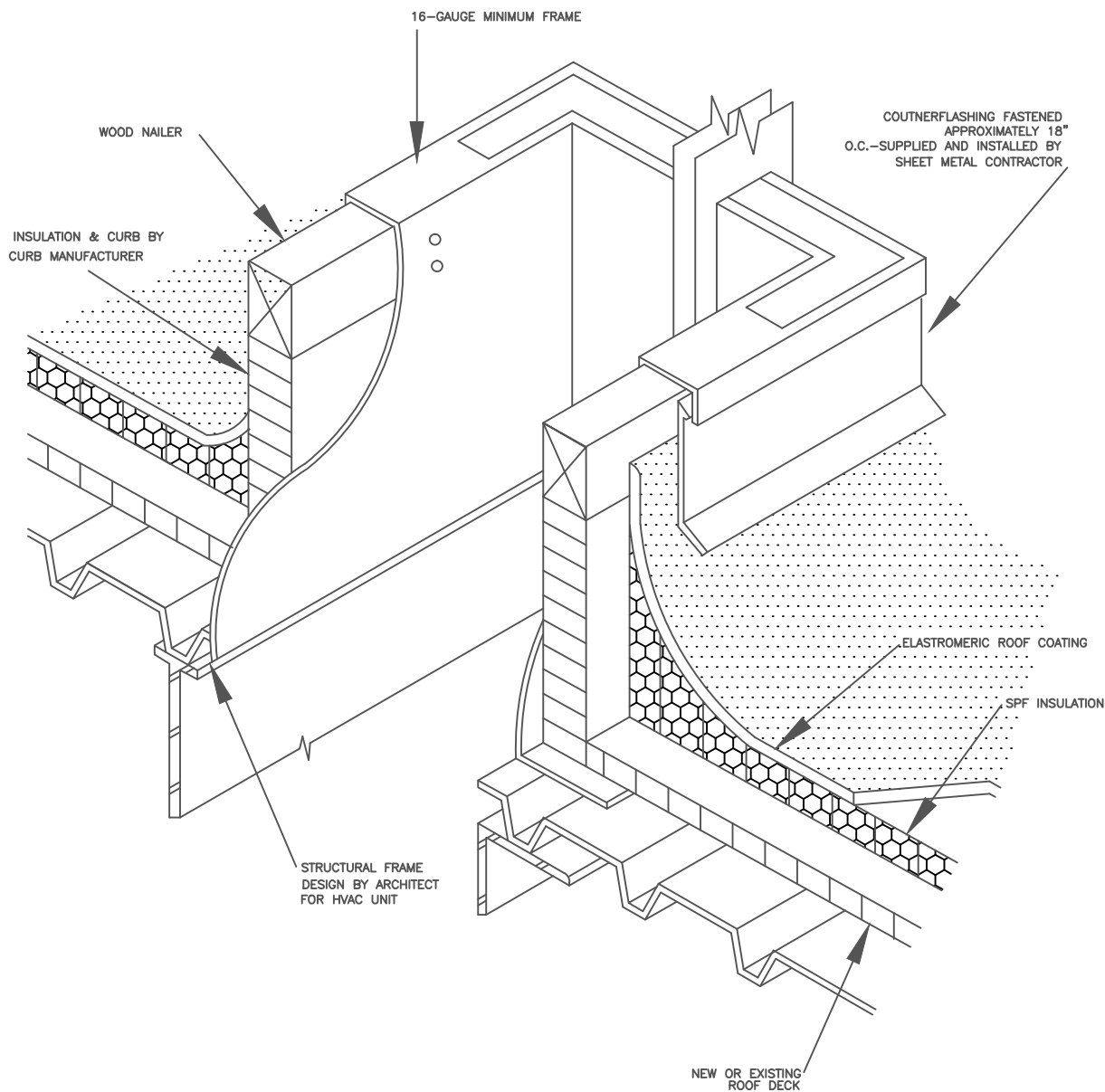
Curb_HVAC_Unit[1]
