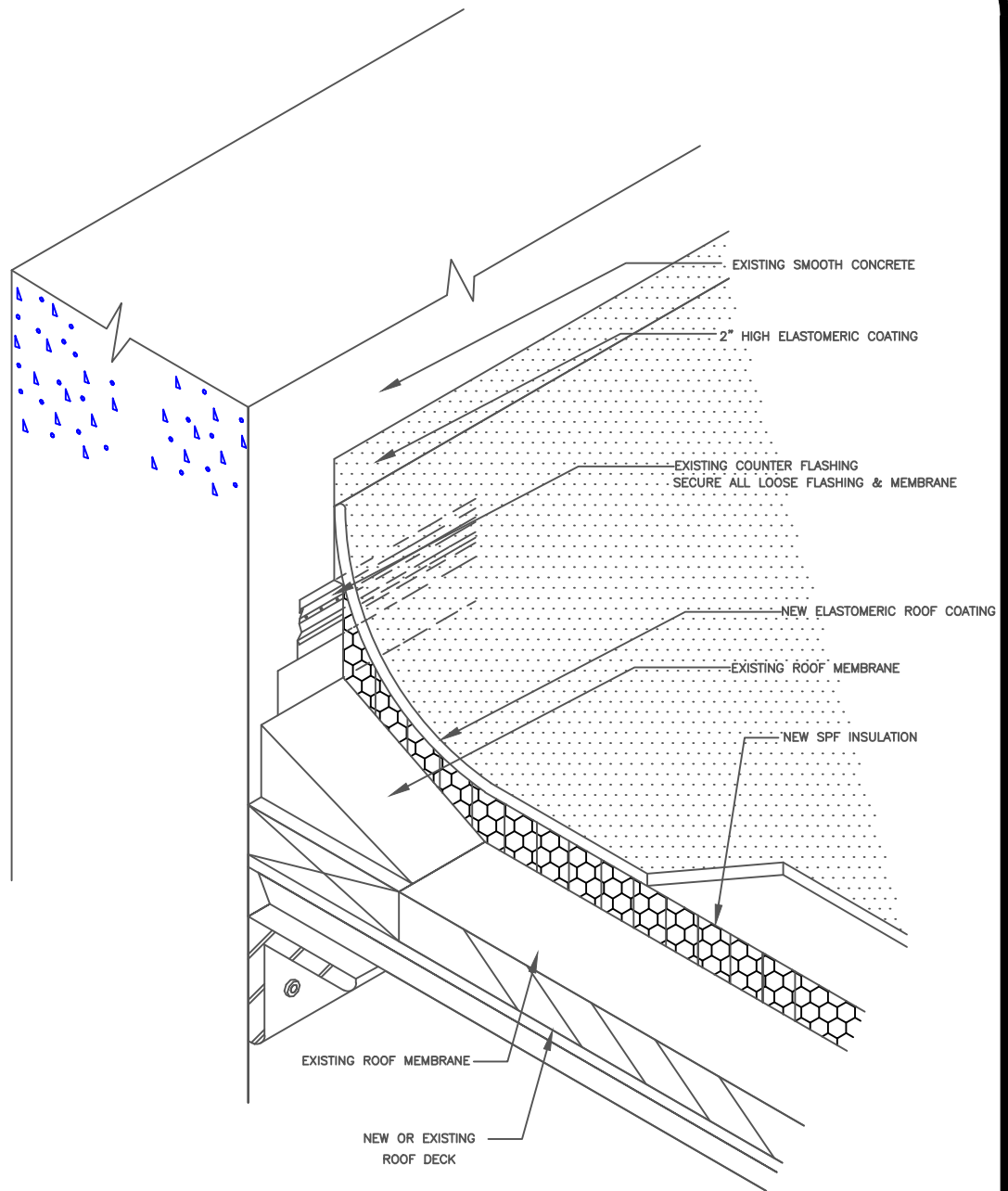
Parapet-ExistingWall-1
