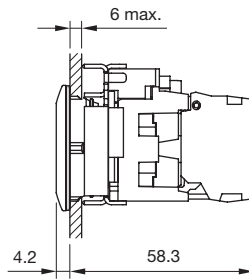
轮廓, 齐平设计 指示灯/按钮开关
