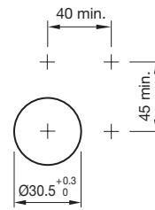
安装图, 齐平设计
