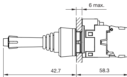
拨动杆
