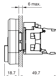
双按钮
