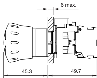
急停开关
