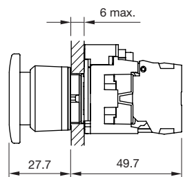
蘑菇头按钮
