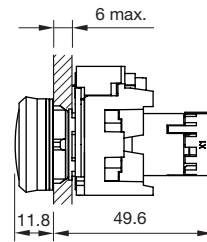
蜂鸣器
