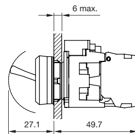
拨动开关
