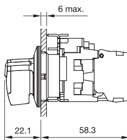
选择开关
