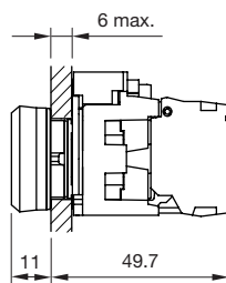
轮廓, 凸起设计 指示灯
