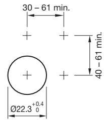
安装图, 凸起设计
