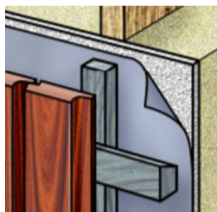
Afbeelding 7 Afgeschuinde achterregel (Bron: Centrum Hout, 2018)
