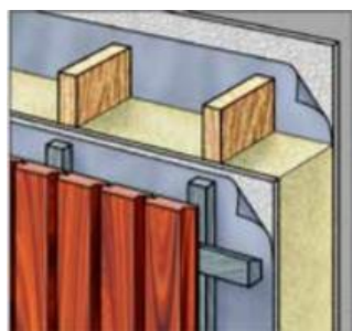
Afbeelding 6 - Dubbel regelwerk (Bron: Centrum Hout, 2018)
