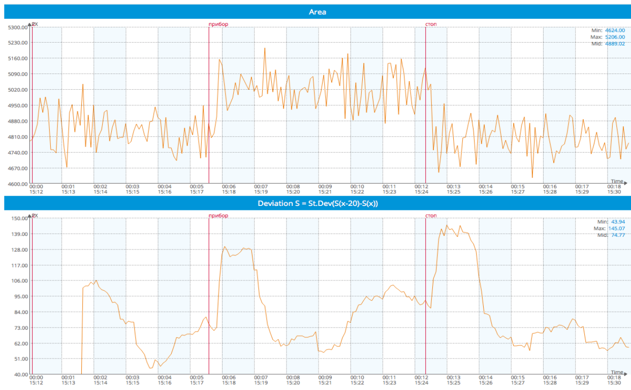
Exemplo 1: Resposta da água a campos eletromagnéticos de alta frequência (o gerador é ligado e desligado).
