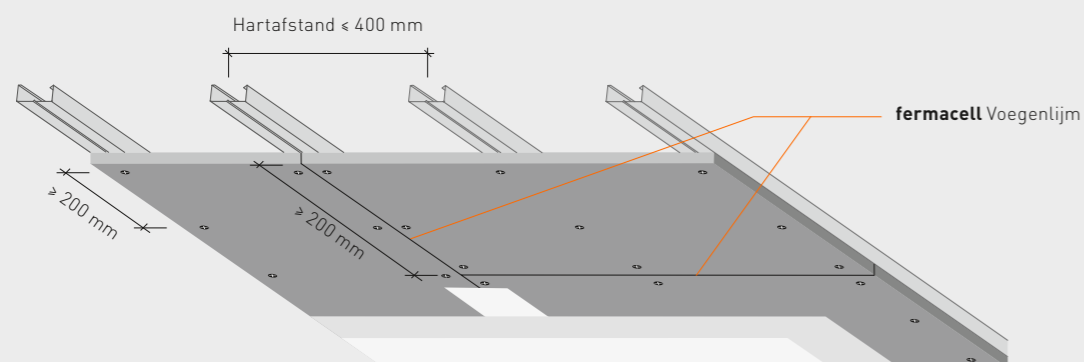
Uitvoering zonder zichtbare plaatnaden
