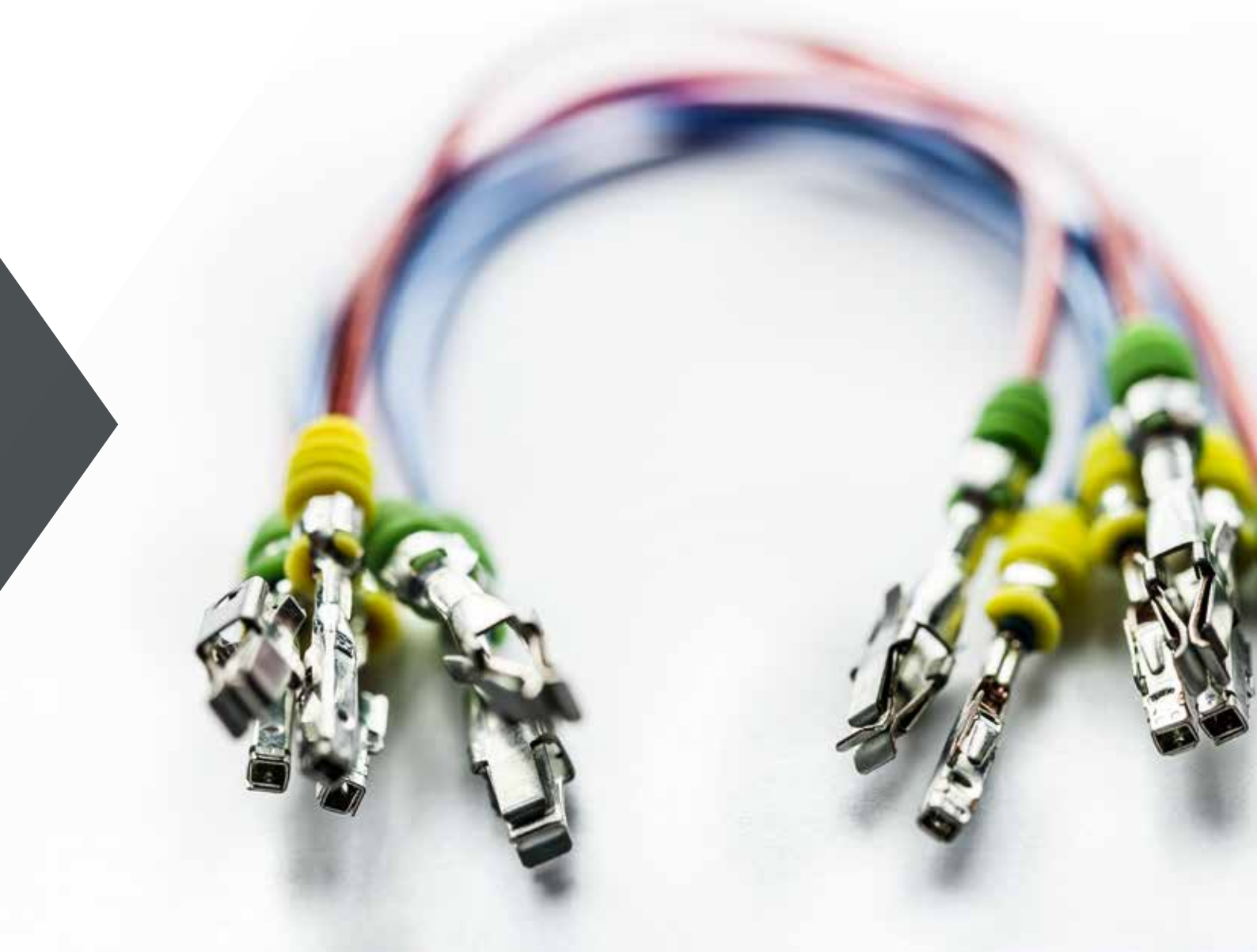
两端压接和两端雨塞插入
