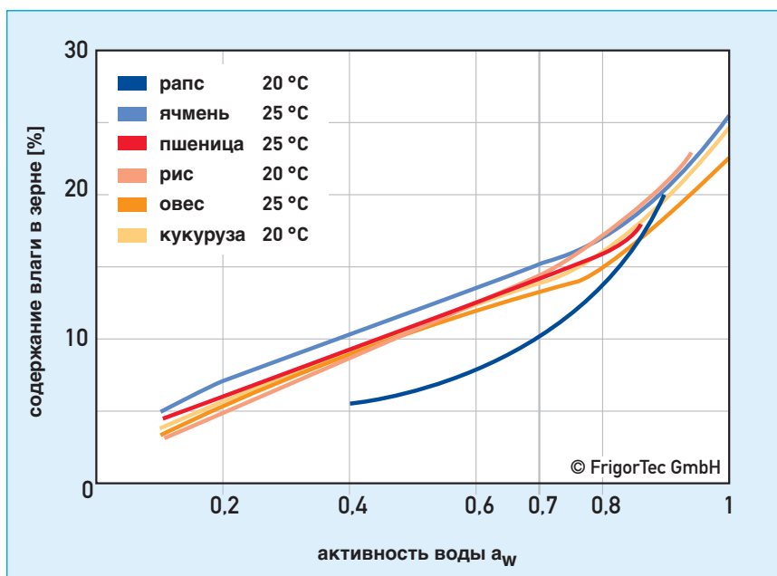
9 Изотермы сорбции различных видов зерна и рапса
