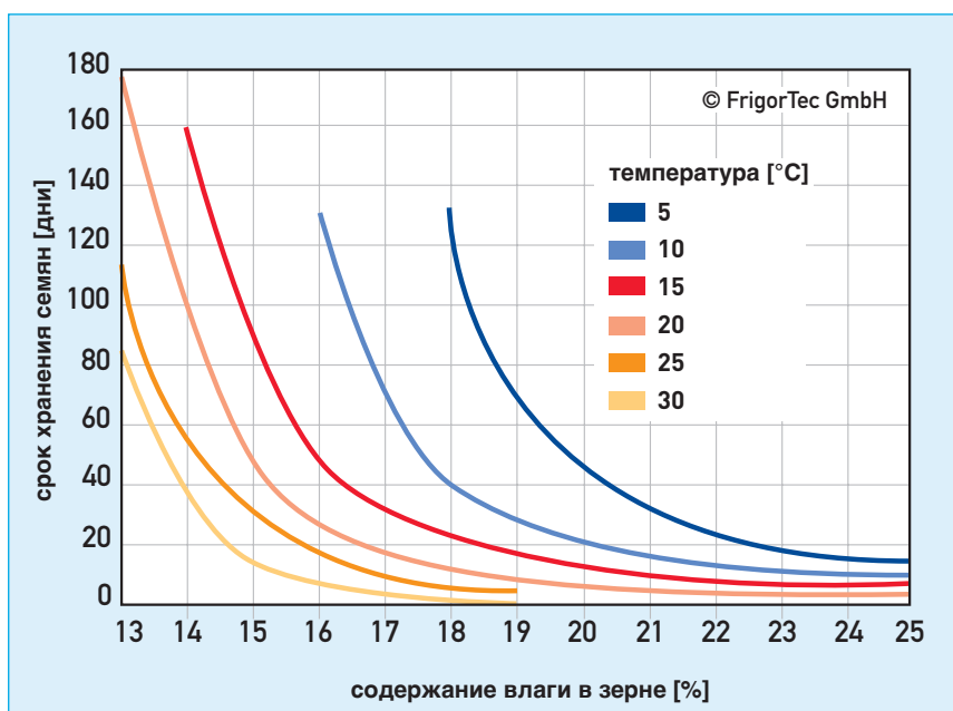
12 Допустимый срок хранения посевного зерна по Agera (13)
